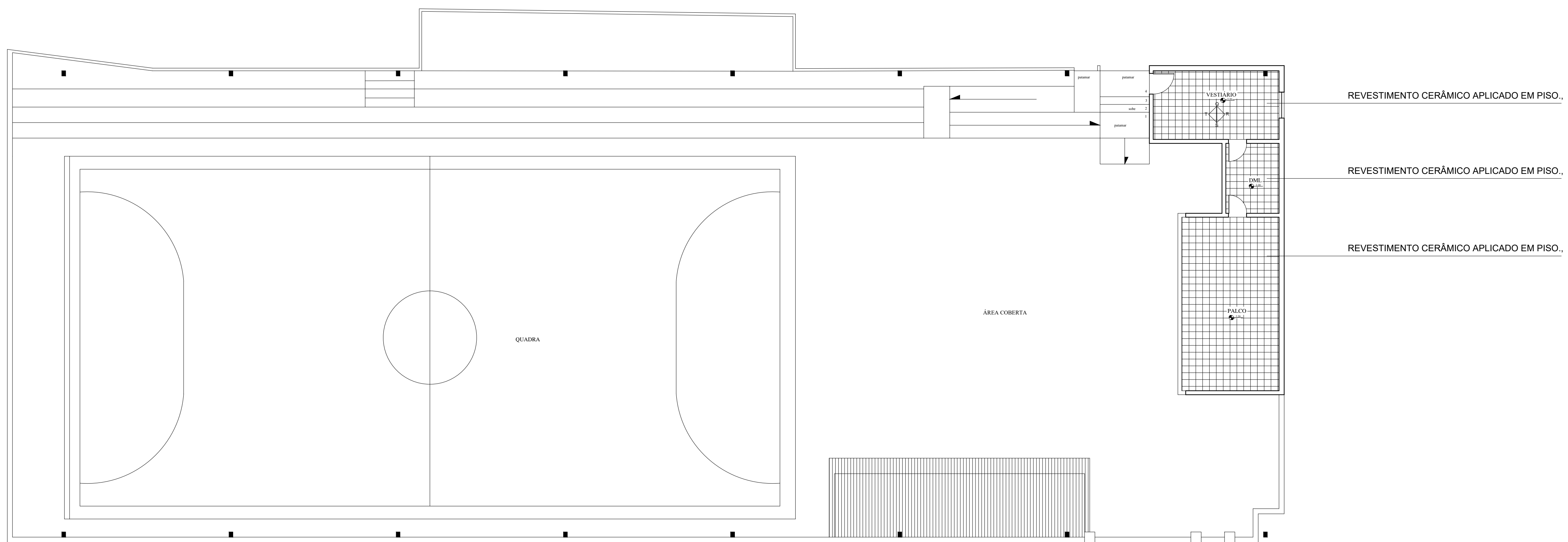
02 | PLANTA DE REFORMA PRIMEIRO PAVIMENTO ESC: 1/100
