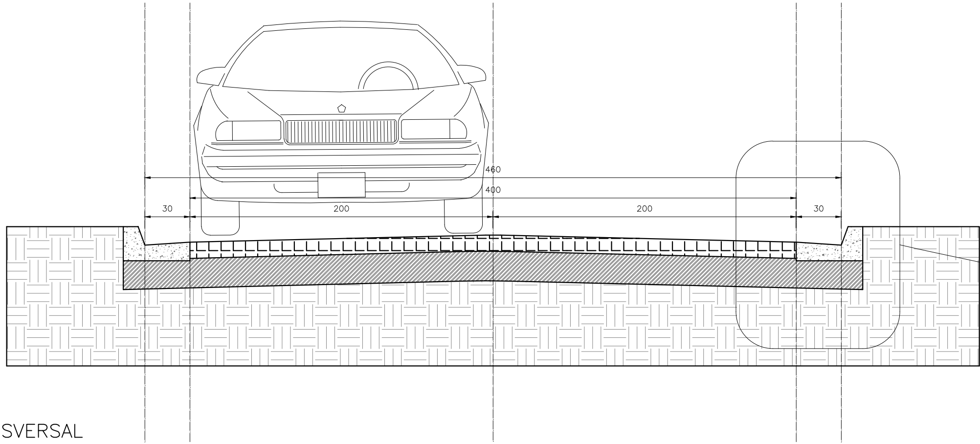
04 | SEÇÃO TRANSVERSAL ESC: 1/25
