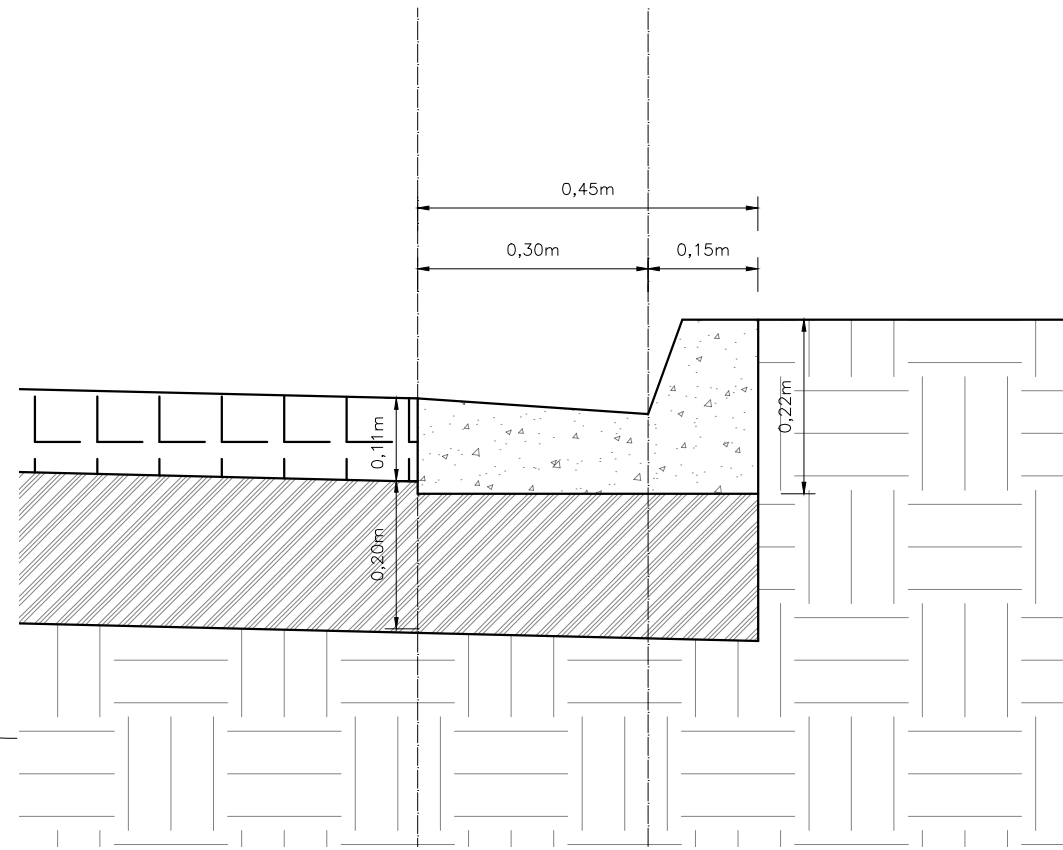
03 | DET. SARJETA ESC: 1/10
