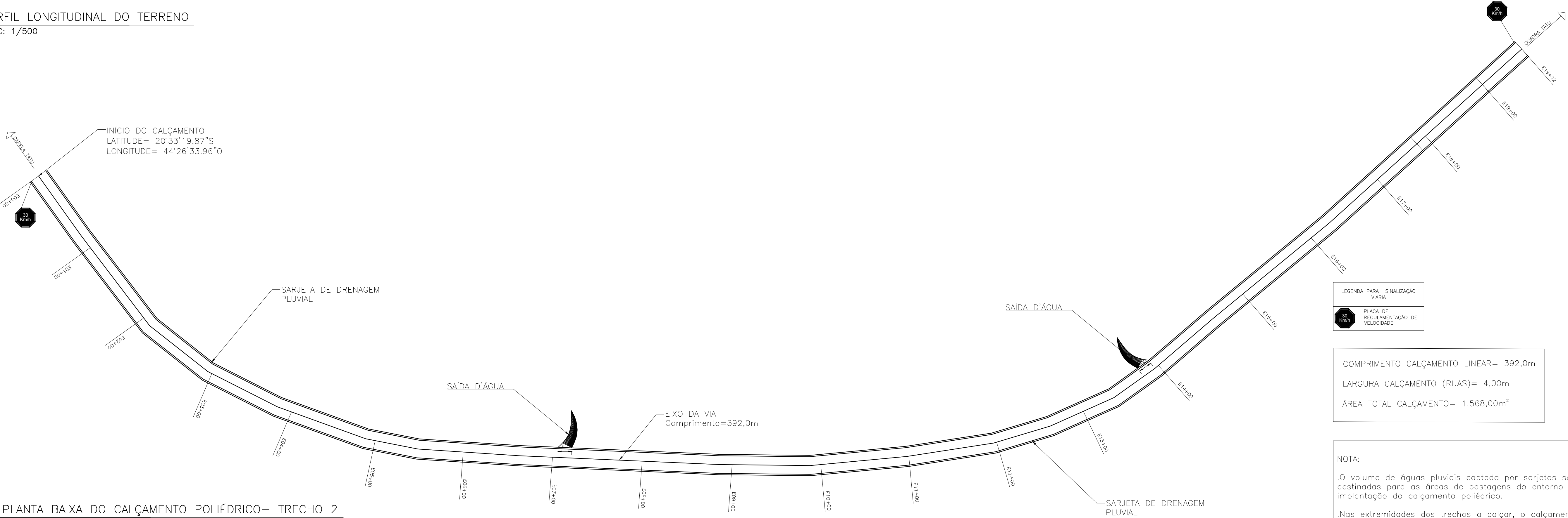
01 | PLANTA BAIXA DO CALÇAMENTO POLIÉDRICO – TRECHO 2 ESC: 1/500
