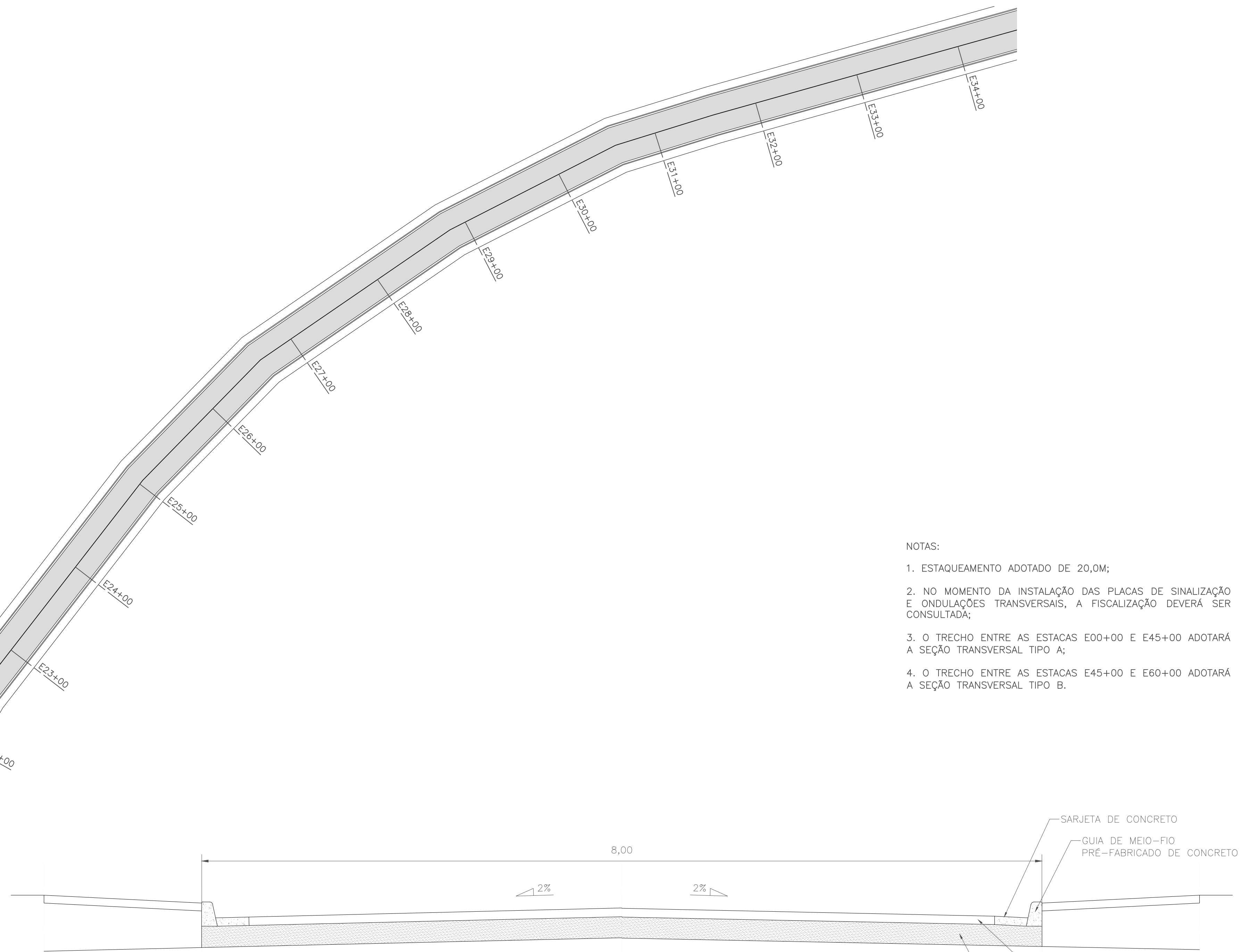
03 SEÇÃO TRANSVERSAL TÍPICA A ESC: 1/25
