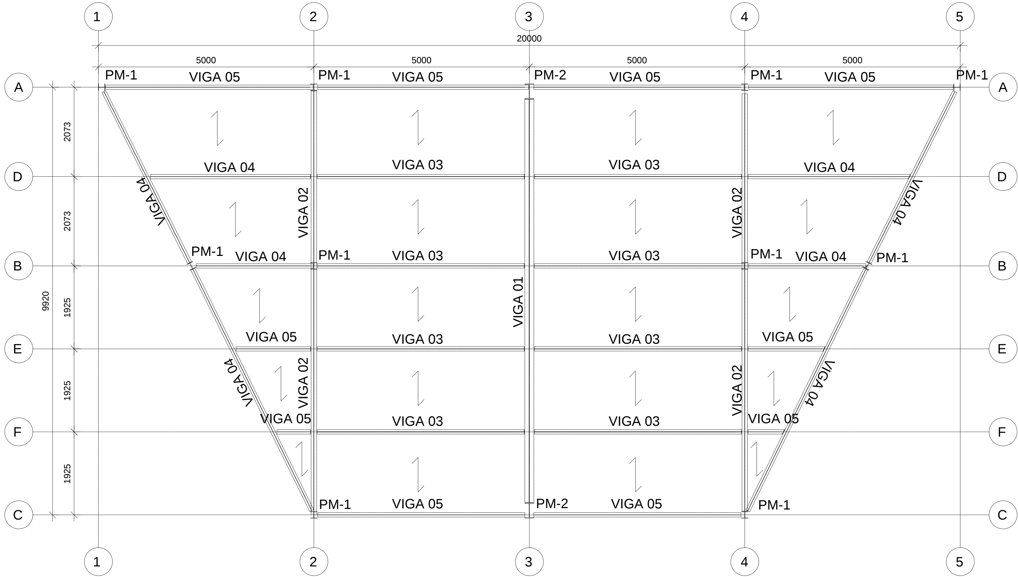
PLANTA DE FÔRMA NIVEL 794,45 ESC: 1/50
