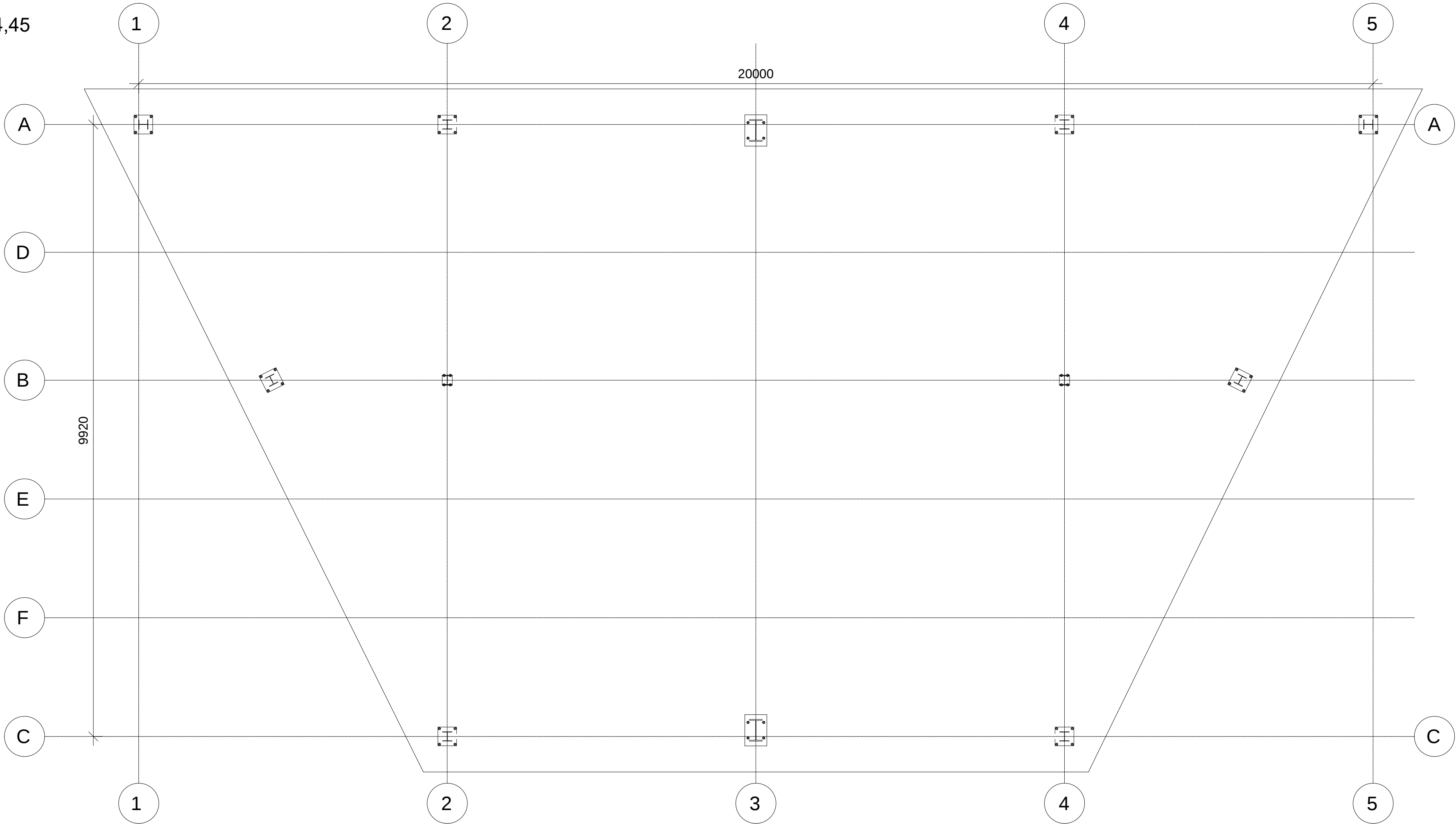
PLANTA DE FÔRMA NIVEL 791,45 ESC: 1/50
